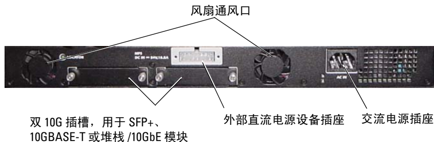
图 1-10. PC7048R 背面板
